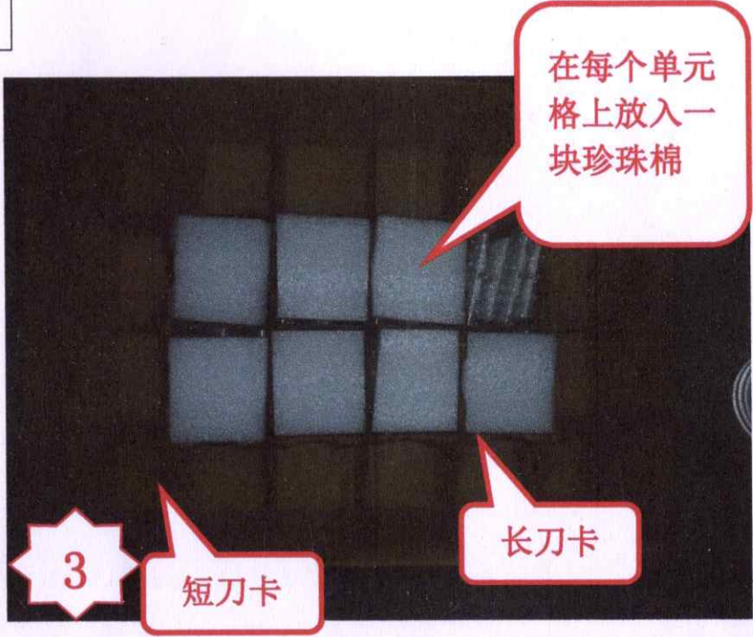
图三, 将 PA603 按照每层 24 格, 每格 4 个, 每箱两层的方式包装, 在每个格子上面放一块珍珠棉, 同时在底层, 中层, 顶层各放一块隔板, 共 3 块隔板。
